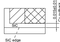
Detail:E
