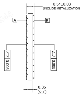
Detail:E
