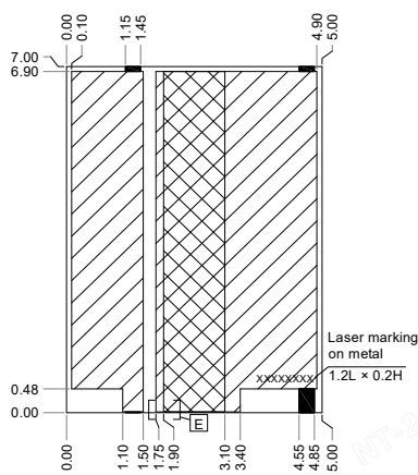
A-side
